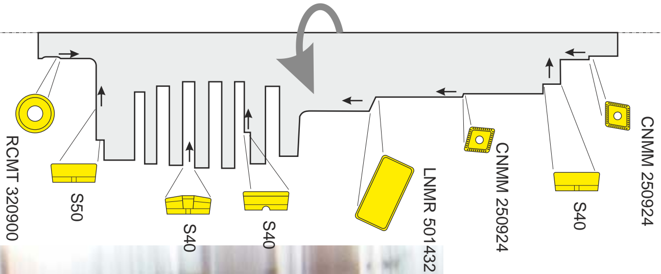
Auswahl geeigneter Schneidplatten Samples of suitable cutting inserts
